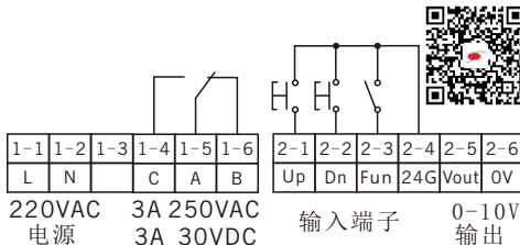
IPC-3SP端子图
