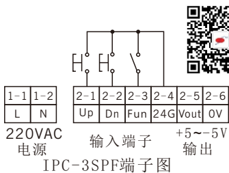
IPC-3SPF端子图
